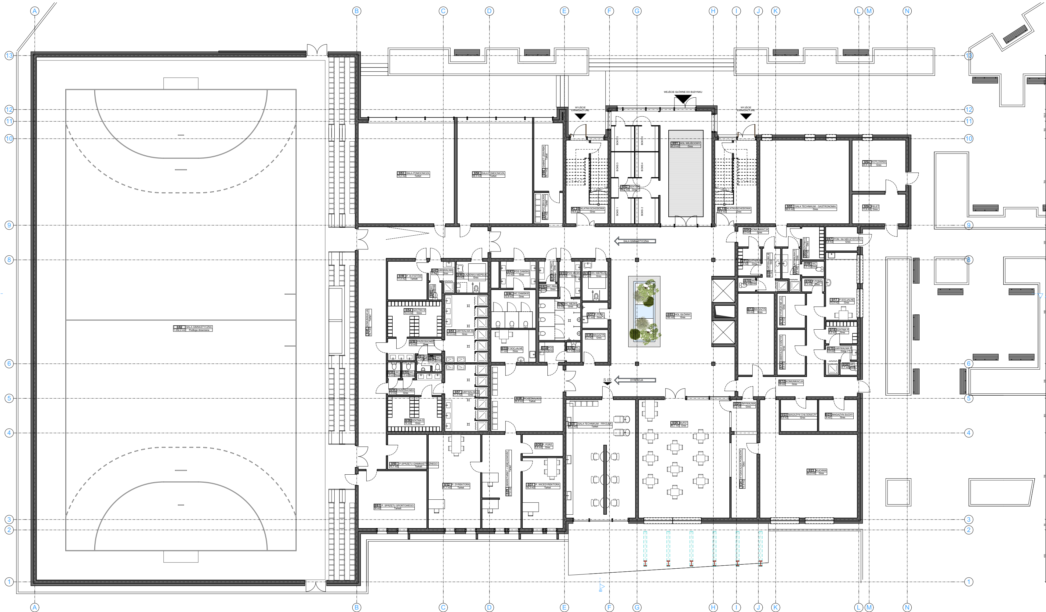
RZUT PRZYZIEMIA POZIOM ± 0
